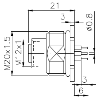
Version mit Lötkontakten / version with soldering contacts
