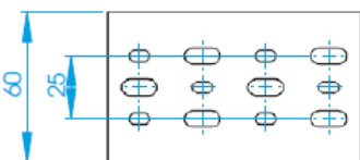
VK 60mm Breite/Width/Largeur
